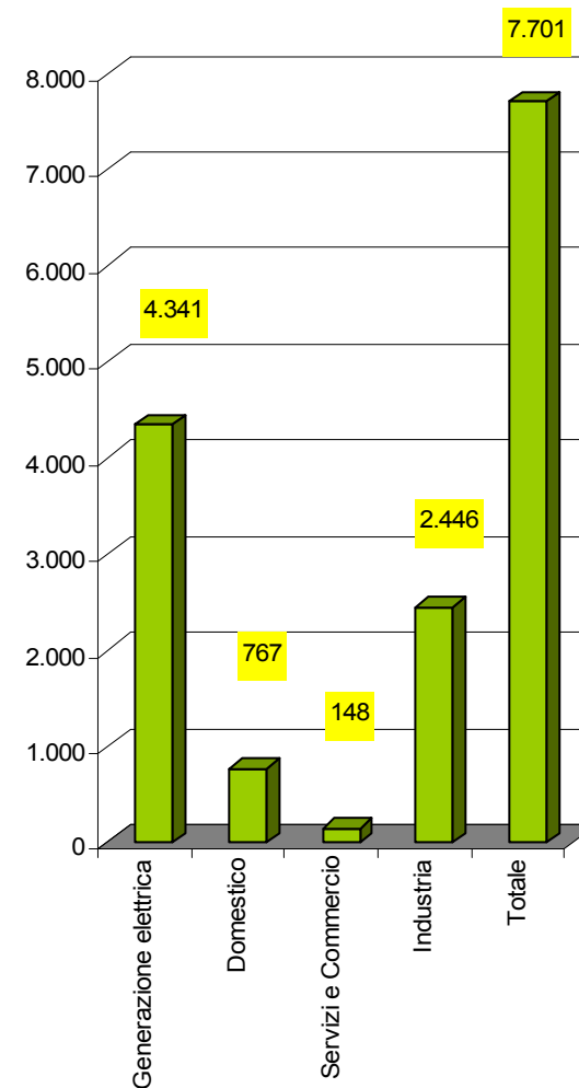
SICILIA GAS NATURALE CONSUMI ENERGETICI PER SETTORE STIMA EMISSIONI DI CO2 ANNO 2007 Migliaia di tonnellate
