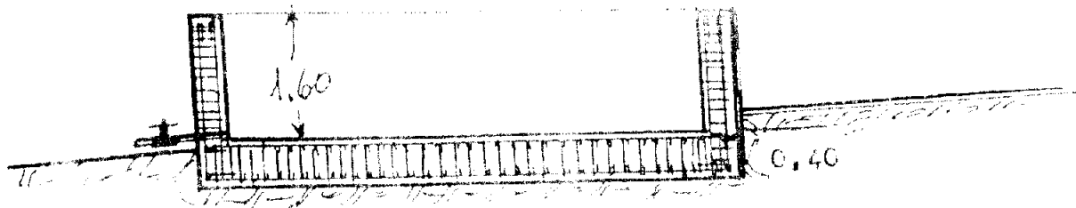
Sezione A-A
