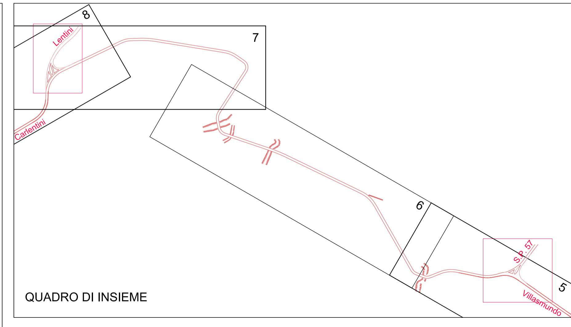
SVINCOLO S.P. 95 - S.P. 57 CARLENTINI - VILLASMUNDO - BRUCOLI Scala 1:500
