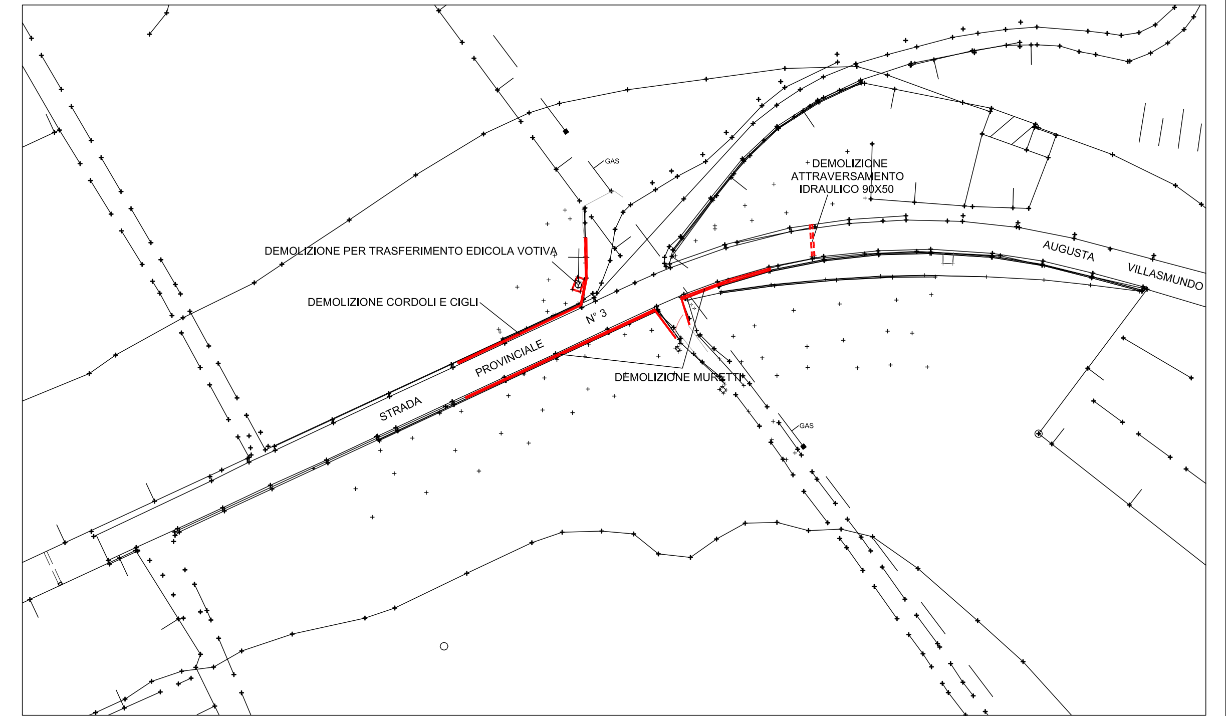
PLANIMETRIA DELLE DEMOLIZIONI 1:1.000
