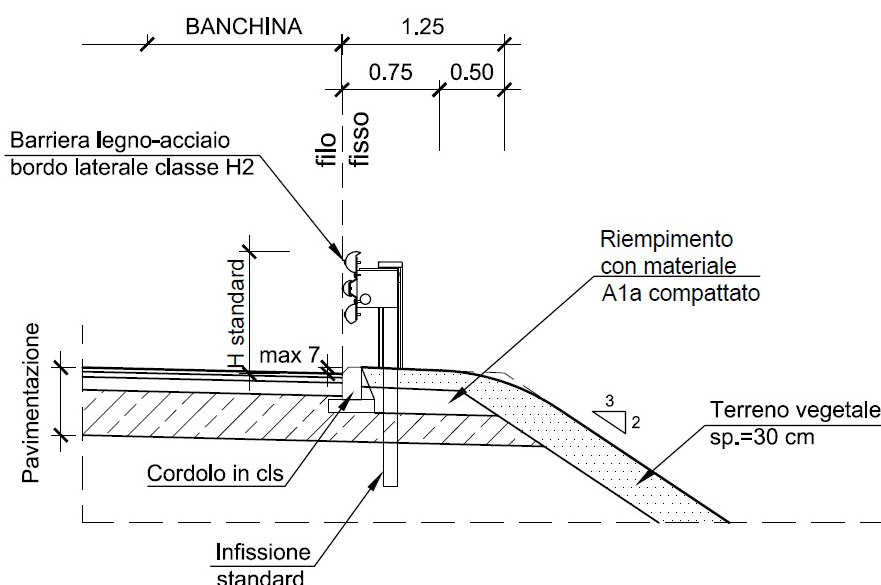
Barriera Anas H2 a bordo rilevato
