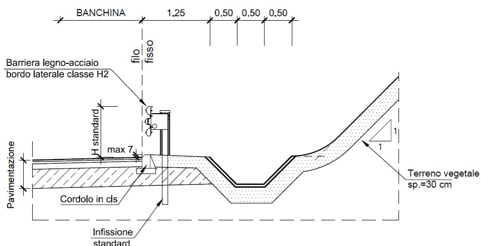
Barriera Anas H2 a bordo trincea
