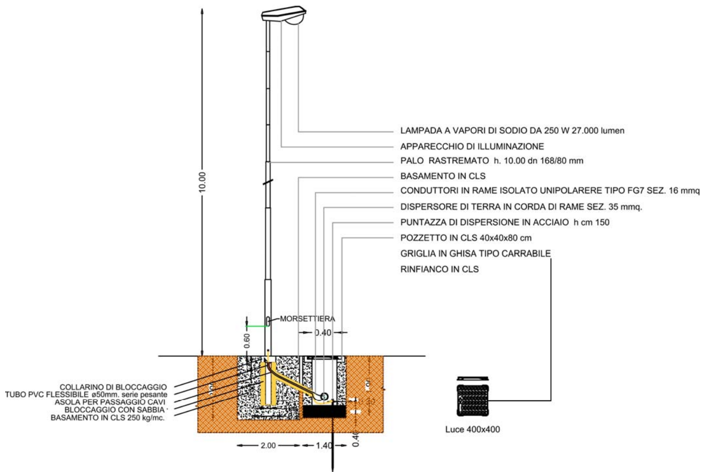
LAMPIONE PER ILLUMINAZIONE STRADALE SCALA 1:10
