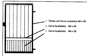
Cancello pedonale in ferro scotolato con cerniere
