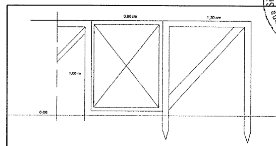
Cancello in ferro e legno e staccionata in legno di castagno
