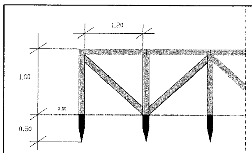
Staccionata in legno di castagno
