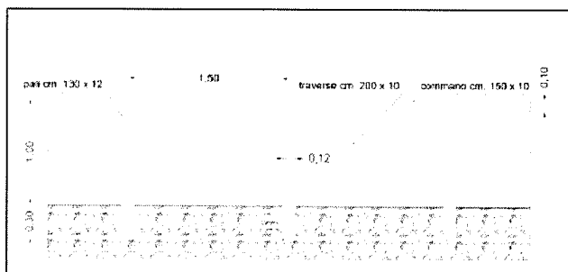
Recinzione in legno di castagno
