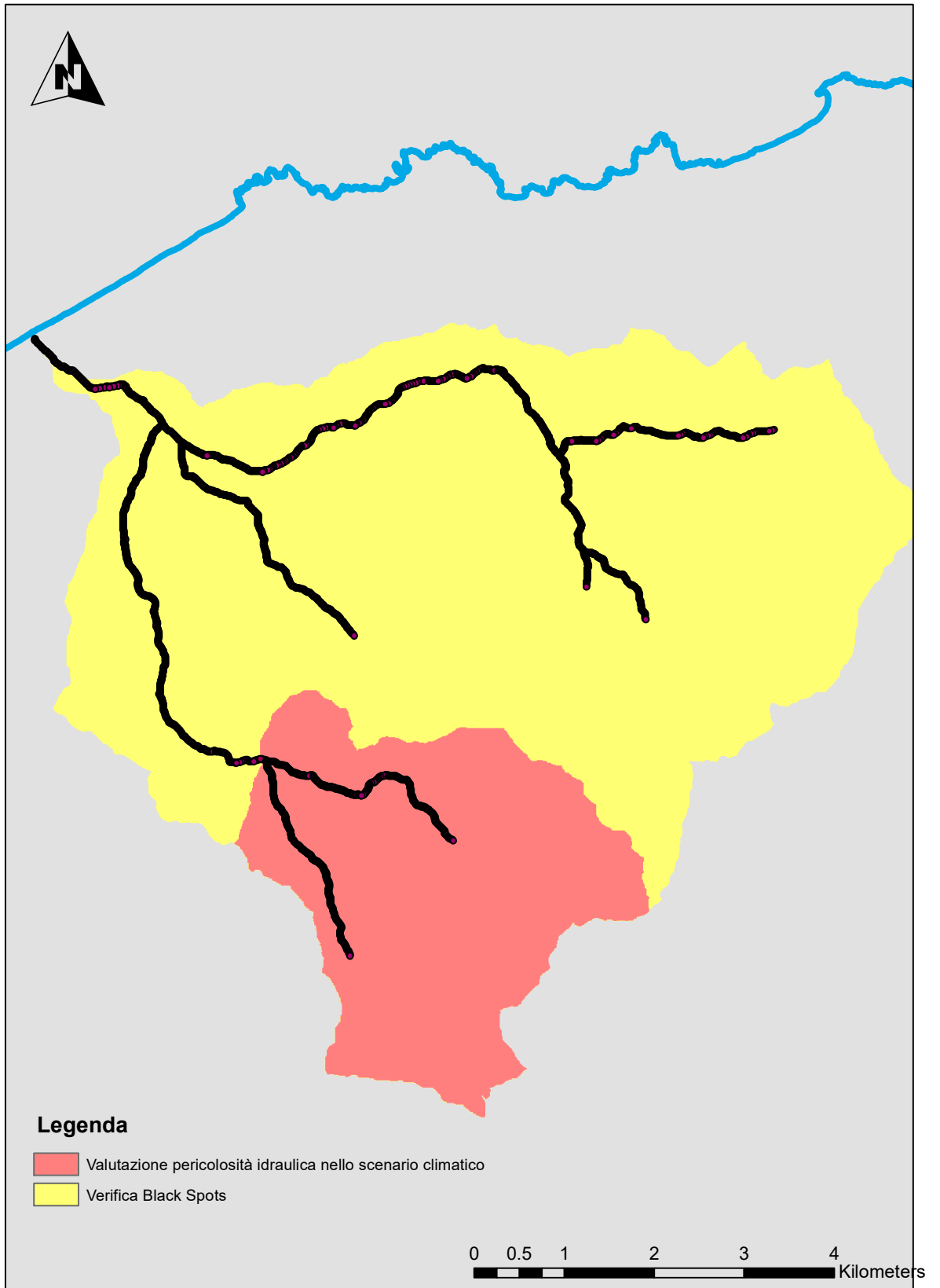
Figura 26 Aree su cui applicare gli interventi di integrazione degli scenari climatici nelle analisi di compatibilità idraulica
