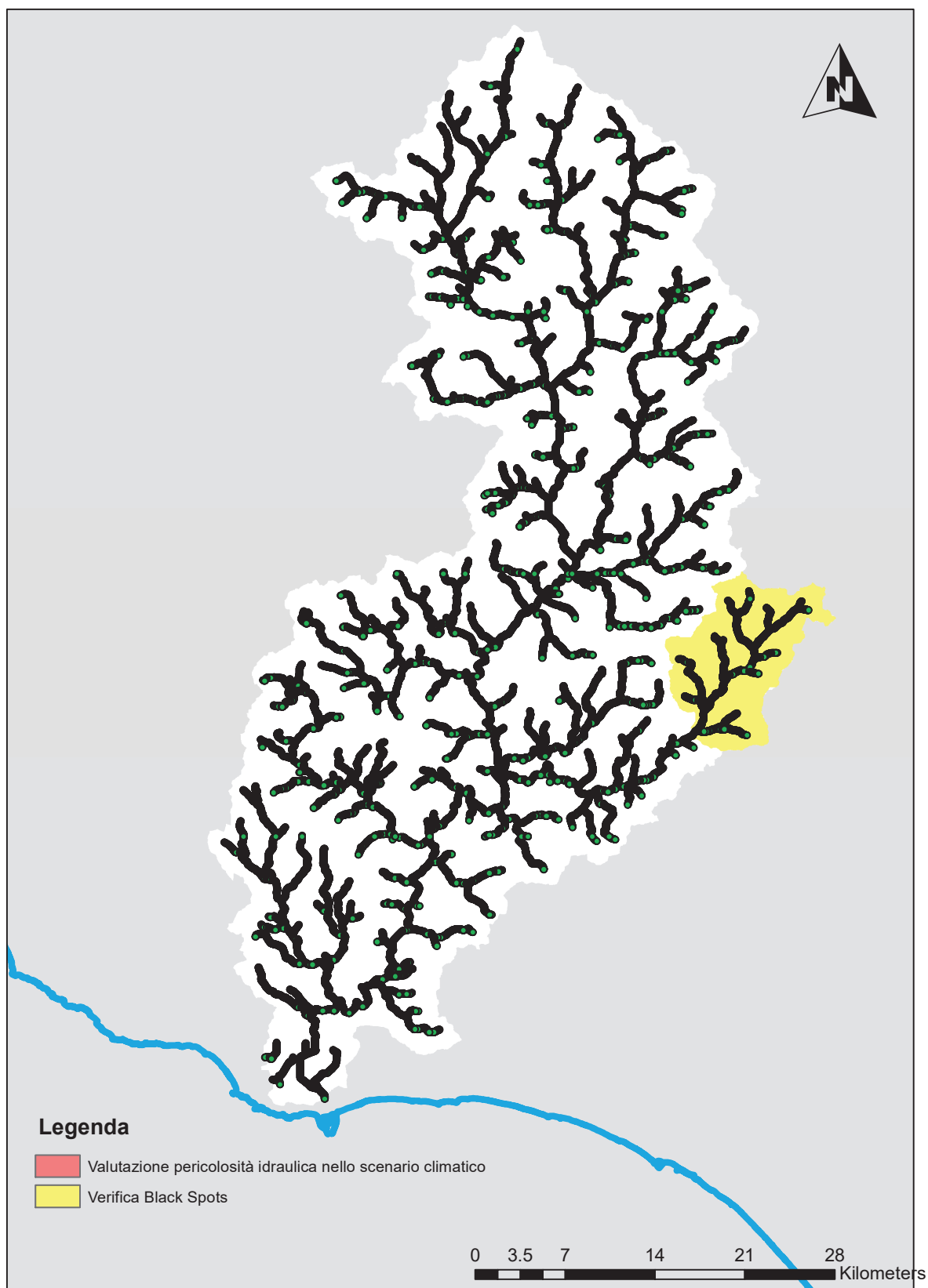
Figura 25 Aree su cui applicare gli interventi di integrazione dei cambiamenti climatici nelle analisi di compatibilità idraulica
