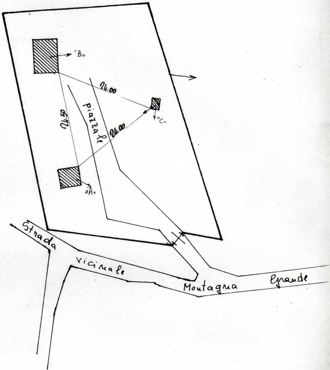
PLANIMETRIA LOTTO INTERESSATO DAI DEPOSITI ESPLOSIVI "A" "B" e "C"
