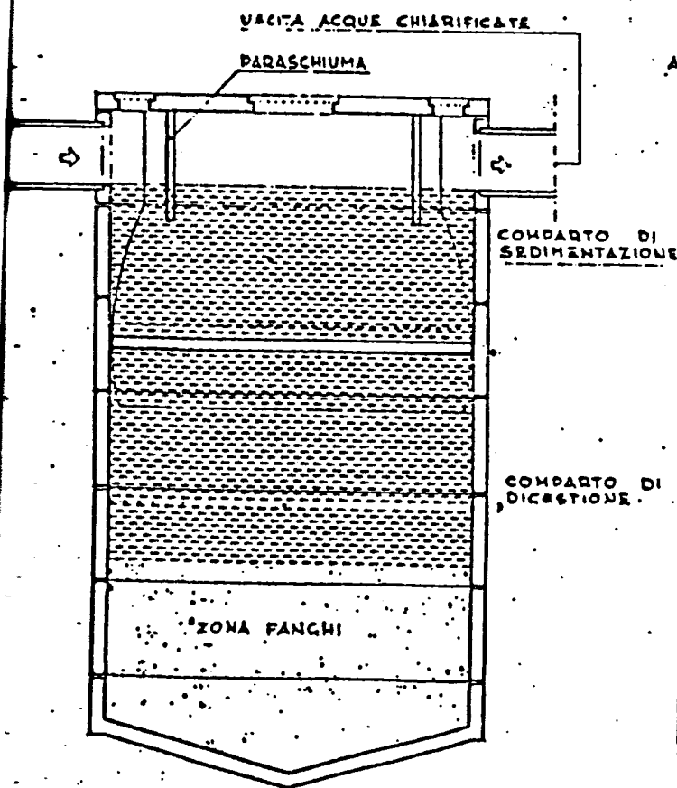
SEZIONE YY
