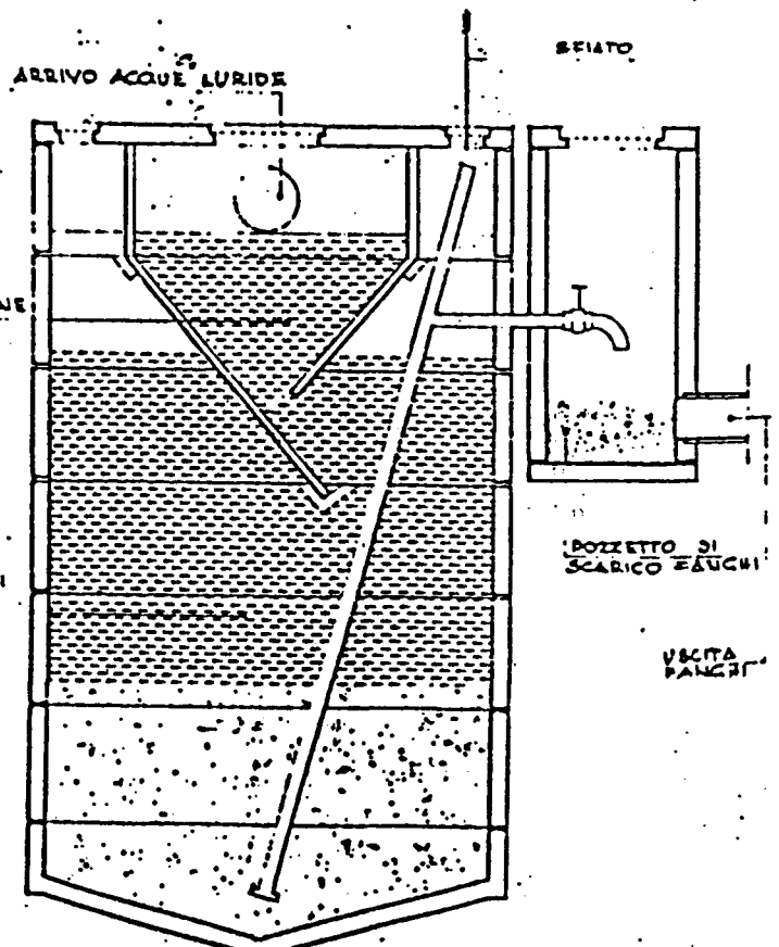
SEZIONE XX
