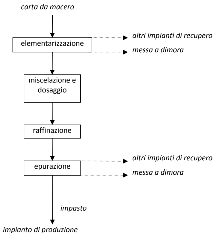
Figura 7.13: Schema tipo del processo produttivo della carta
