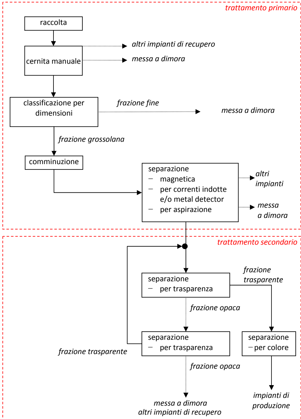
Figura 7.9: Schema tipo di trattamento per il recupero del vetro
