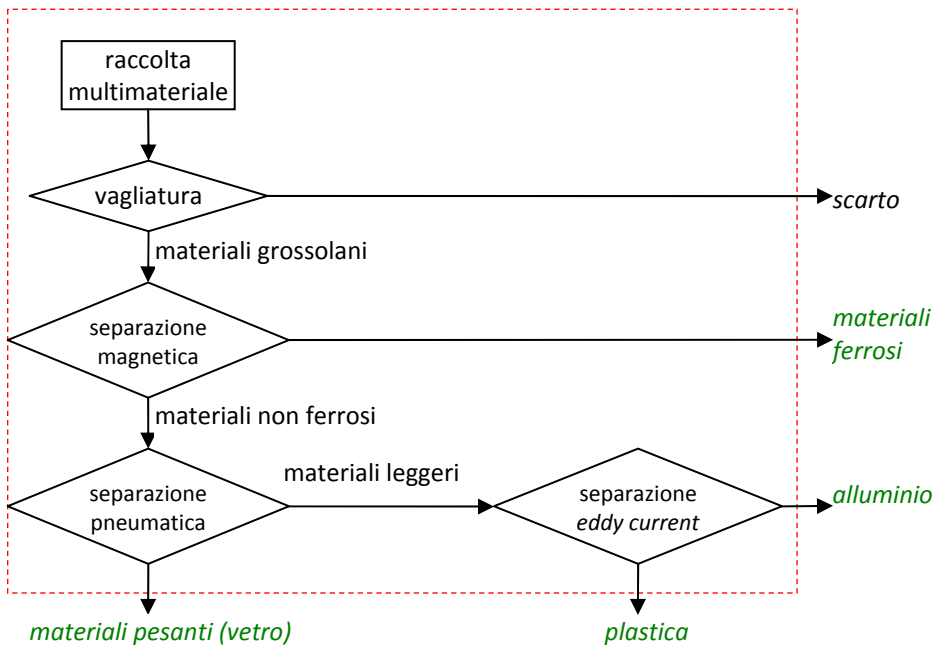
Figura 7.3: Schema di selezione dei rifiuti provenienti da raccolta differenziata multimateriale
