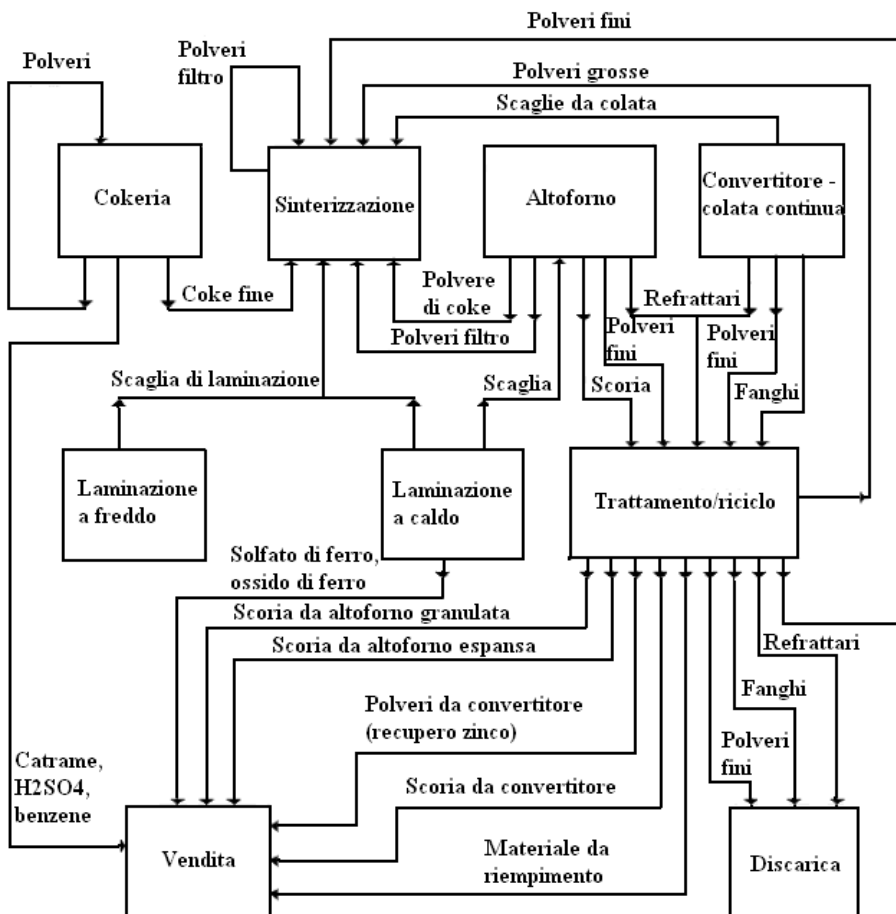
Figura 6.7: Schema semplificato del flusso dei residui, dei sottoprodotti e dei rifiuti in una acciaieria a ciclo integrato
