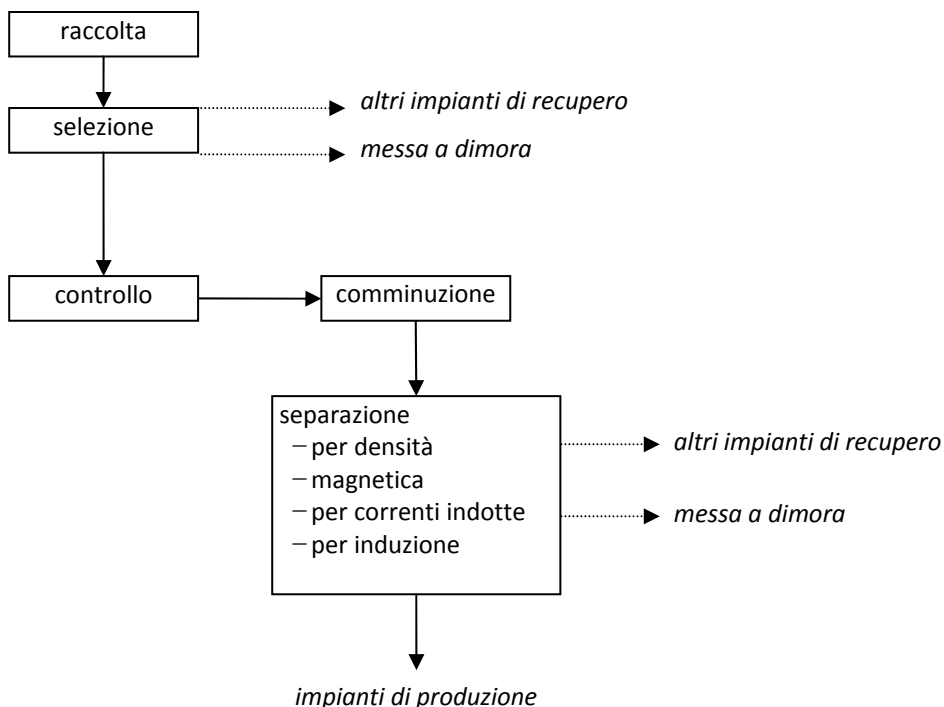
Figura 7.10: Schema tipo di trattamento per il recupero dei metalli
