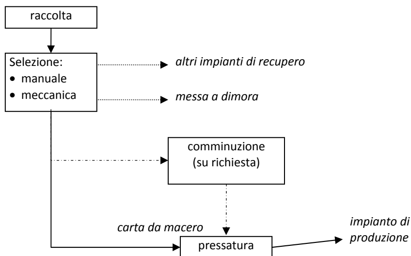
Figura 7.12: Schema tipo per la raccolta e la lavorazione della carta da macero
