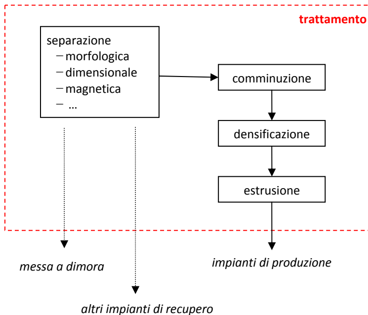
Figura 7.6: Schema tipo di trattamento per il recupero della plastica
