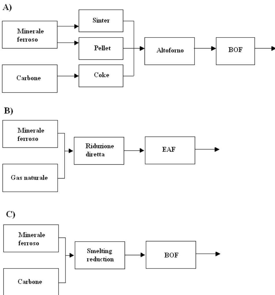
Figura 6.6: Schemi di produzione dell'acciaio mediante il ciclo integrato (A), per riduzione diretta (B) e per smelting reduction (C). (BOF = Basic Oxygen Furnace ; EAF = Electric Arc Furnace )
