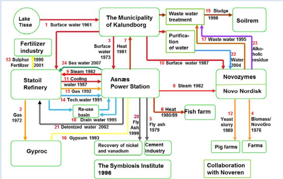
Figura 3.2: La rete degli scambi e delle relazioni operanti nell'area industriale di Kalundborg (2007), Fonte: Jørgen Christensen, 2006
