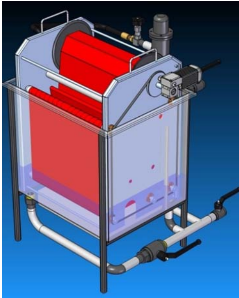
Figura 9.3: Apparecchiatura prototipale OBEM per tintura tessuti in piano
