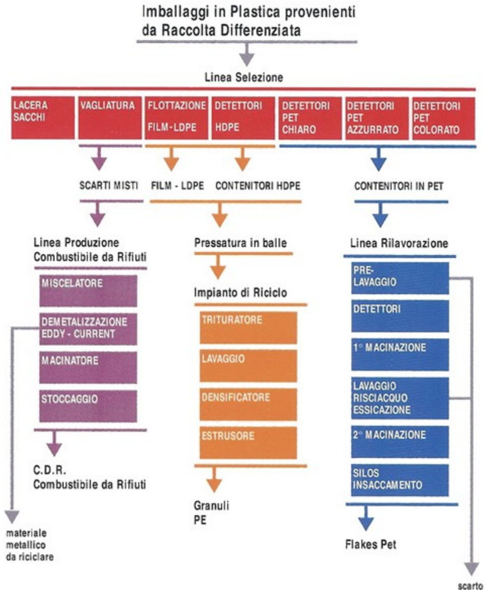
Figura 7.8: Schema del processo di trattamento per il recupero della plastica – Montello SpA, stabilimento di Montello (BG)
