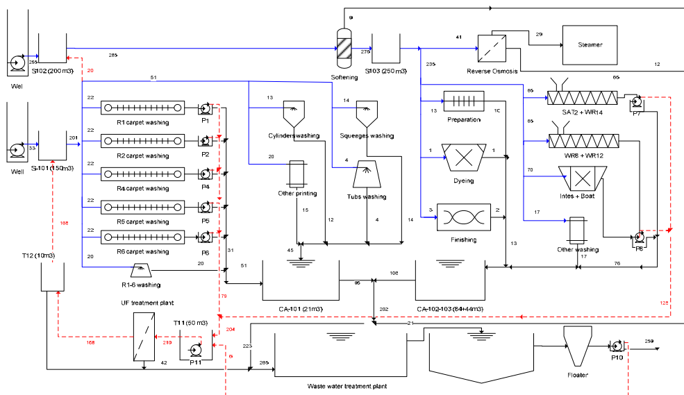
Figura 9.2: Schema concettuale impianto BATTLE
