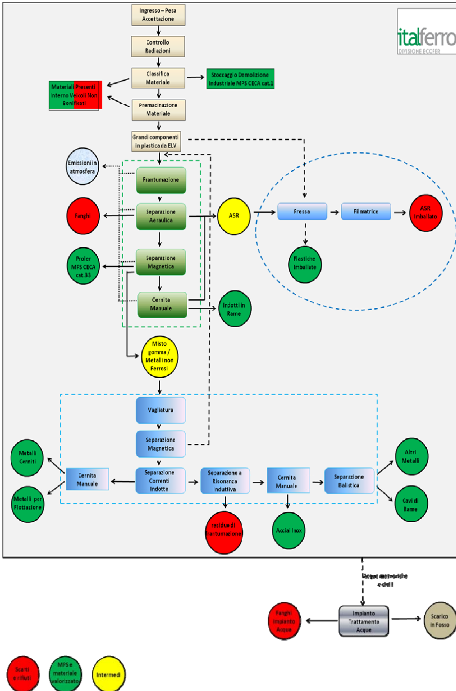
Figura 7.11: Schema del processo di trattamento per il recupero dei metalli – Gruppo Fiori, stabilimento Italferro di Roma
