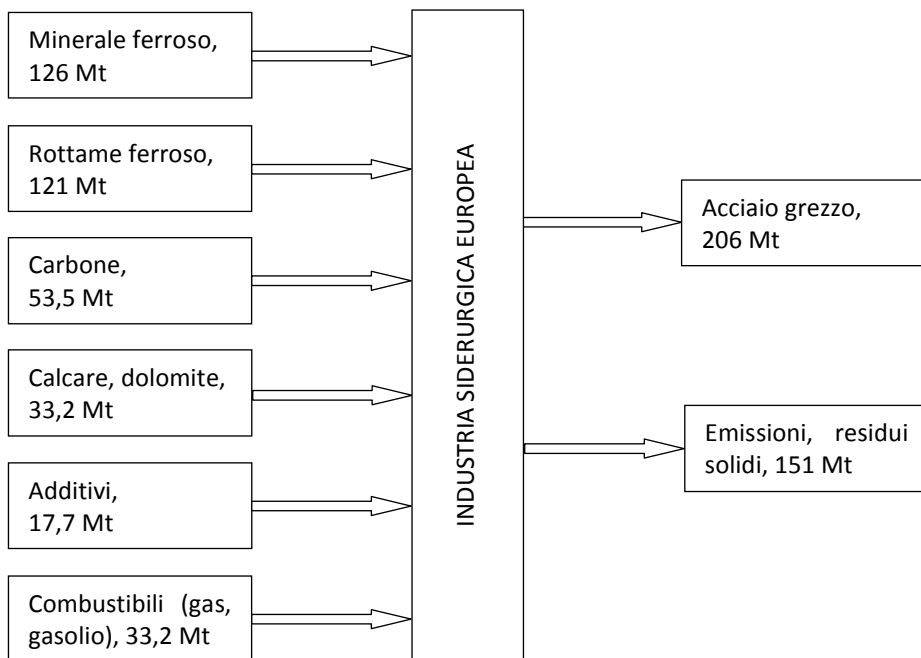
Figura 6.5: Flussi di massa nell'industria siderurgica europea (EU-27) nel 2006
